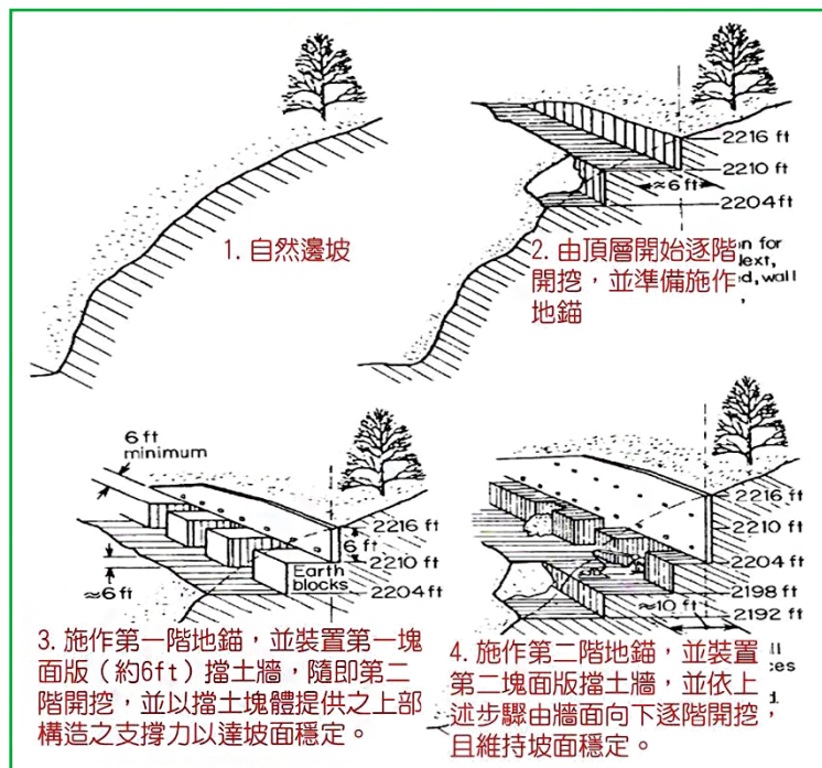
巴西地錨工法施工步驟
